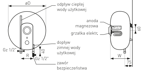
Ogrzewacz nadumywalkowy Mars
